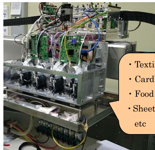
1800mm textile フルカラー印刷装置ヘッド部分
